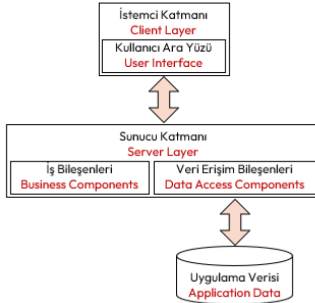
Şekil 19.2: İstemci-Sunucu Mimarisi
